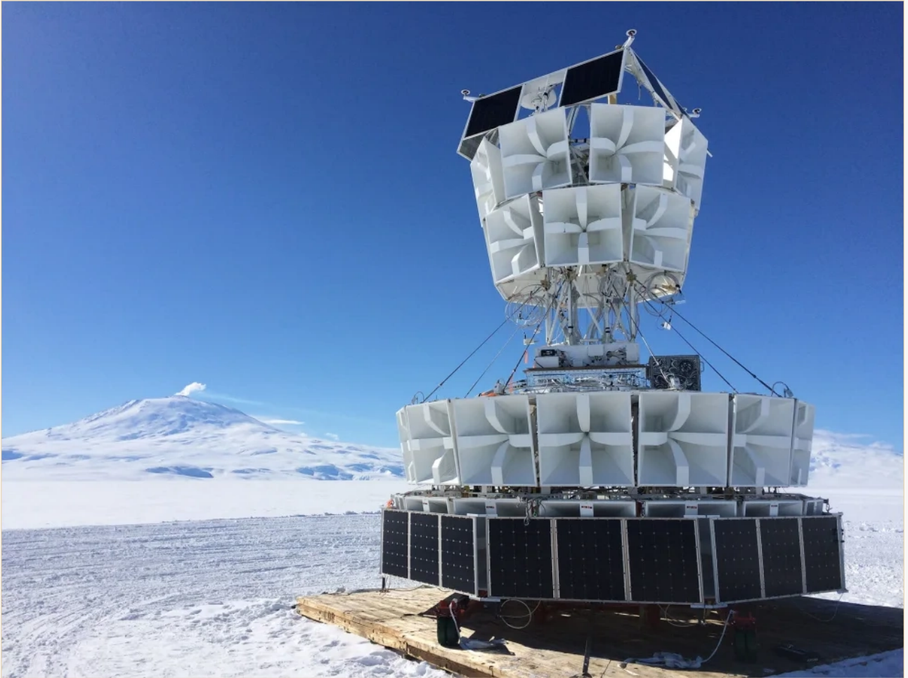
የANITA 48 አንቴናዎች 25 ሜትር ከፍታ ባለው ጎንደላ ላይ ሆነው ወደ አንታርክቲካ በረዶ ወደ ታች ያነጣጥራሉ።
